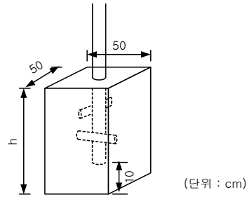
<그림 11> 기초의 규격
