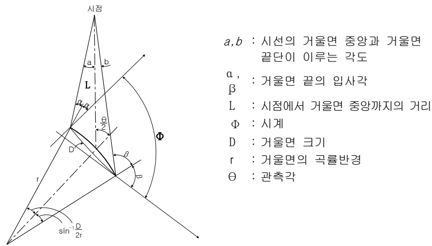
〈그림 8〉 도로반사경의 시계
